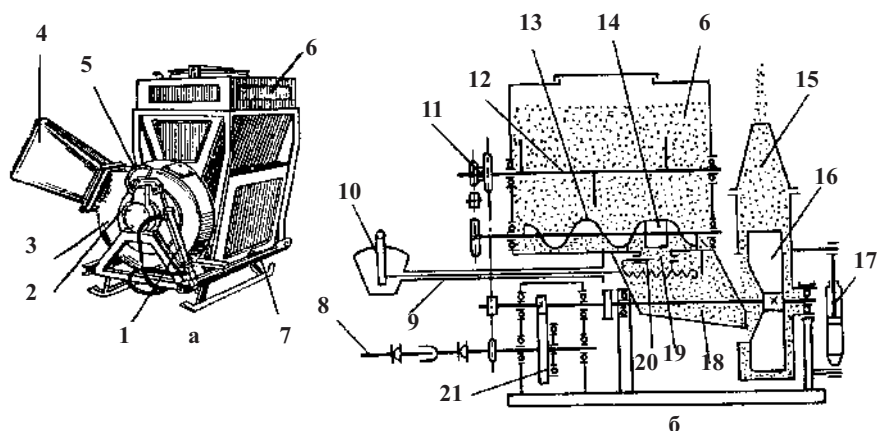
8.3. сурет. ОШУ-50А әмбебап кеңқамтушы бүріккіш:
